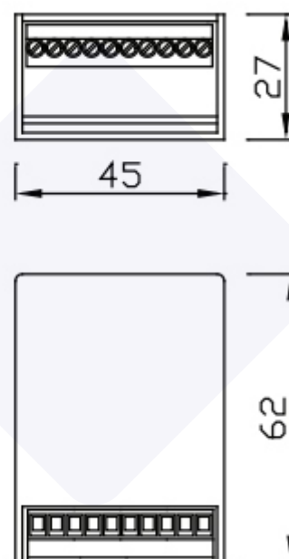
réleový připojovací modul
